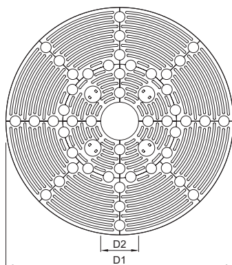
Exempelritning: Typ 44
