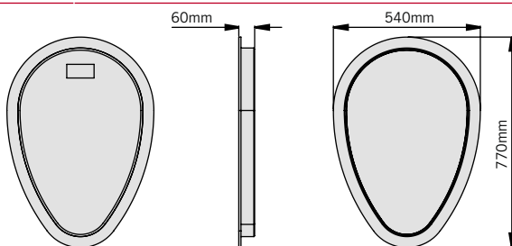
ACO Qmax ® 700 blanking end cap
